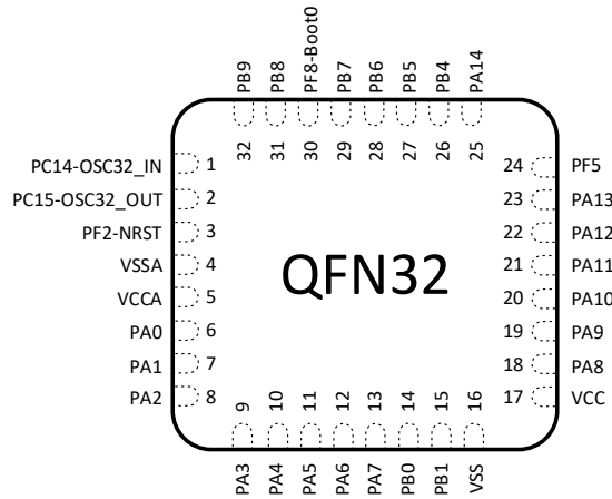
图 3-5 QFN32 PY32F071K1xU Pinout1
