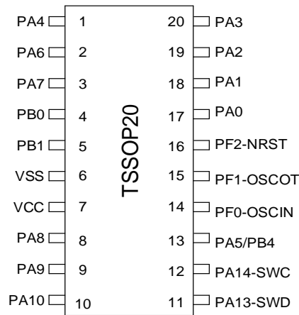
图 3-15 TSSOP20 Pinout4 PY32F030F4xP
