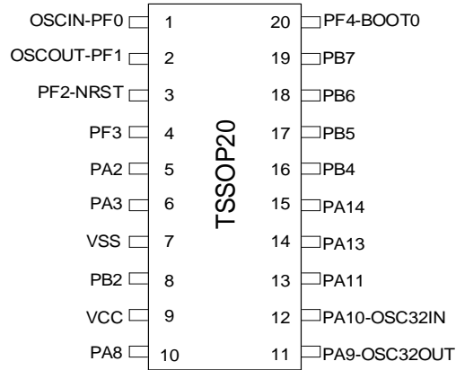
图 3-12 TSSOP20 Pinout1 PY32F030F1xP
