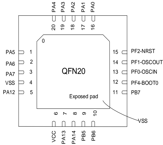
图 3-10 QFN20 Pinout2 PY32F030F2xU / -E
