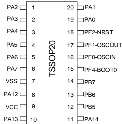
图 3-13 TSSOP20 Pinout2 PY32F030F2xP
