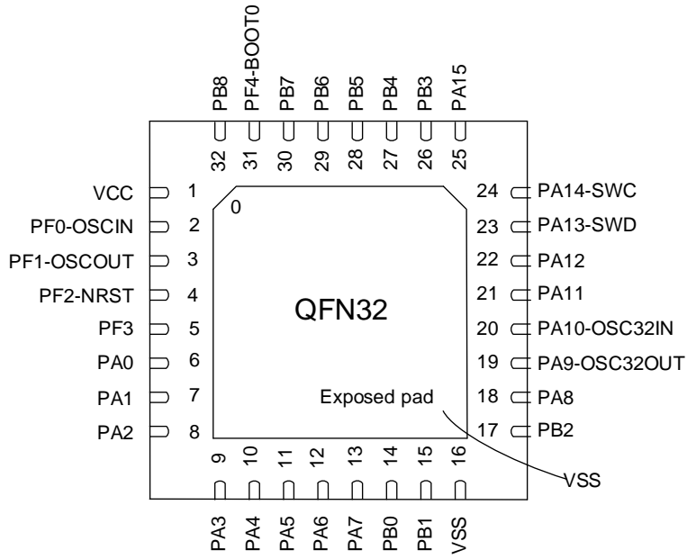
图 3-3 QFN32(5*5) Pinout2 PY32F030K2xU / -E
