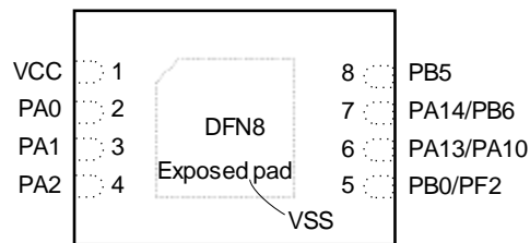
图 3-16 DFN8(1.5*1.5) Pinout1 PY32F030L1xD
