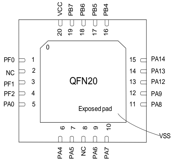
图 3-11 QFN20 Pinout3 PY32F030F3xU
