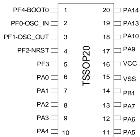
图 3-14 TSSOP20 Pinout3 PY32F030F3xP
