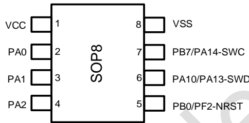
图 3-14 SOP8 PY32F003L2xS
