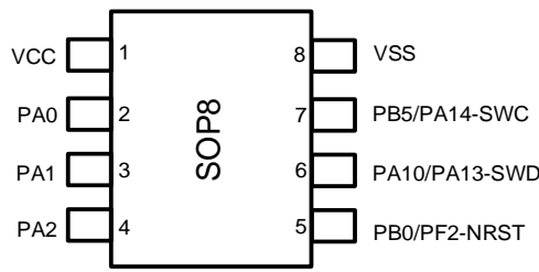
图 3-13 SOP8 PY32F003L1xS
