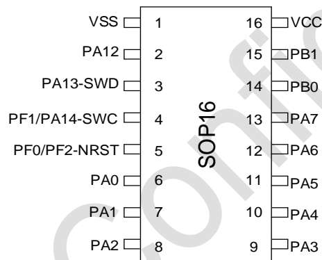
图 3-10 SOP16 Pinout1 PY32F003W1xS / -E
