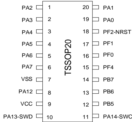
图 3-3 TSSOP20 Pinout1 PY32F003F1xP / -E
