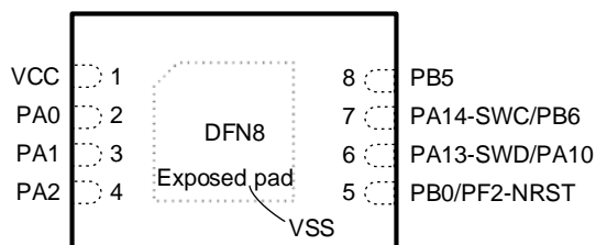
图 3-12 DFN8(3*2) PY32F003L2xD
