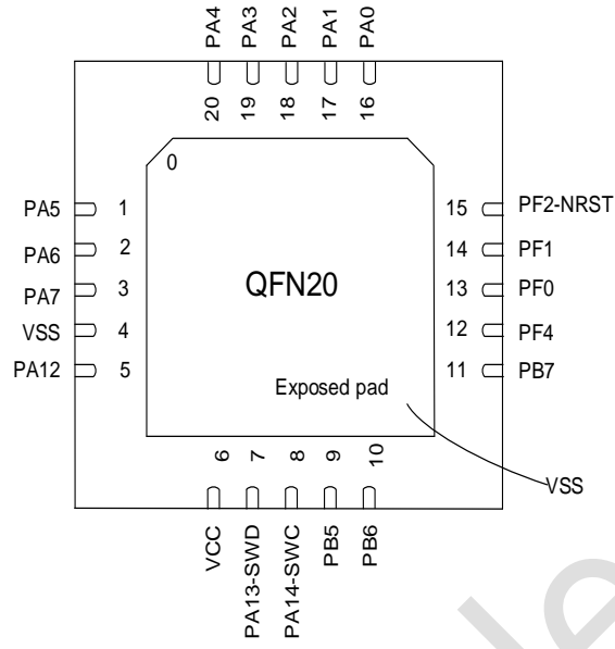
图 3-1 QFN20 Pinout1 PY32F003F1xU
